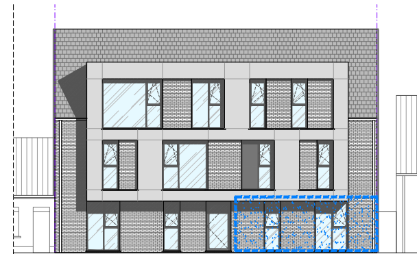
VOORGEVEL
