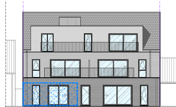
ACHTERGEVEL
