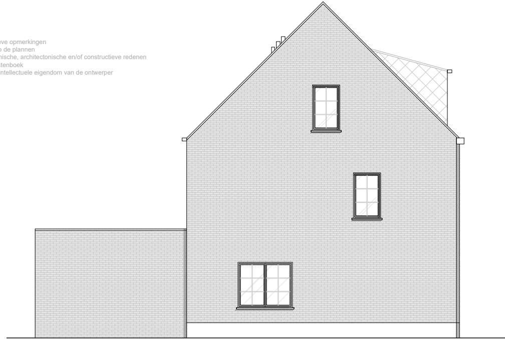
zijgevel
