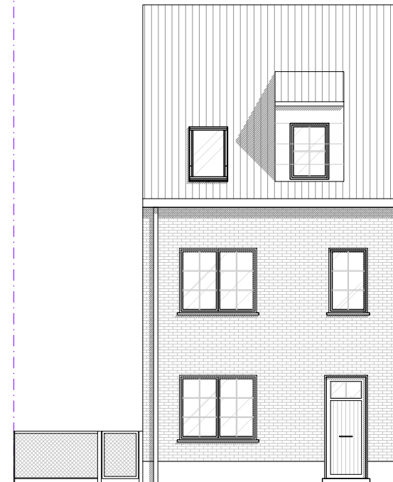
voorgevel
