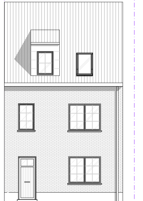
voorgevel
