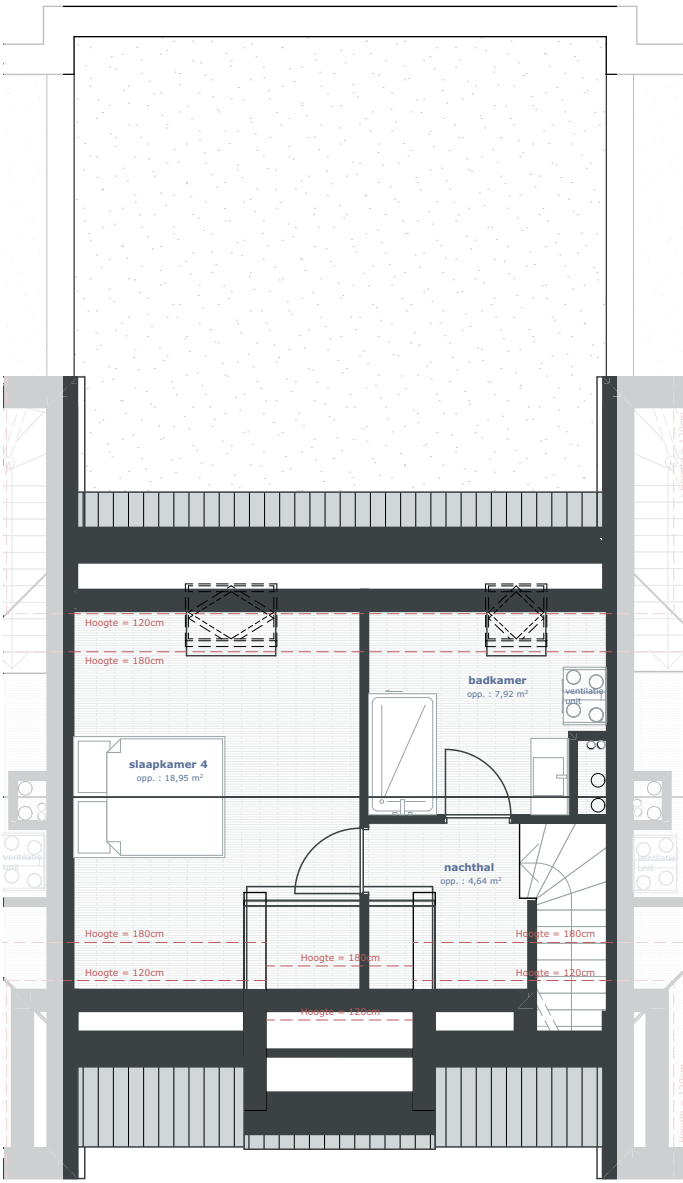
NIVO +2 - 1:100
