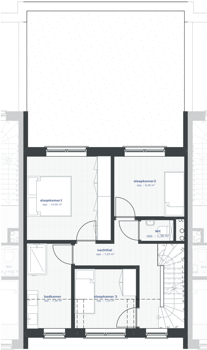
NIVO +1 - 1:100
