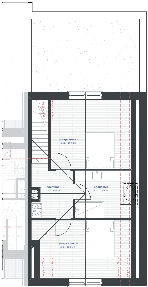
NIVO +2 - 1:100
